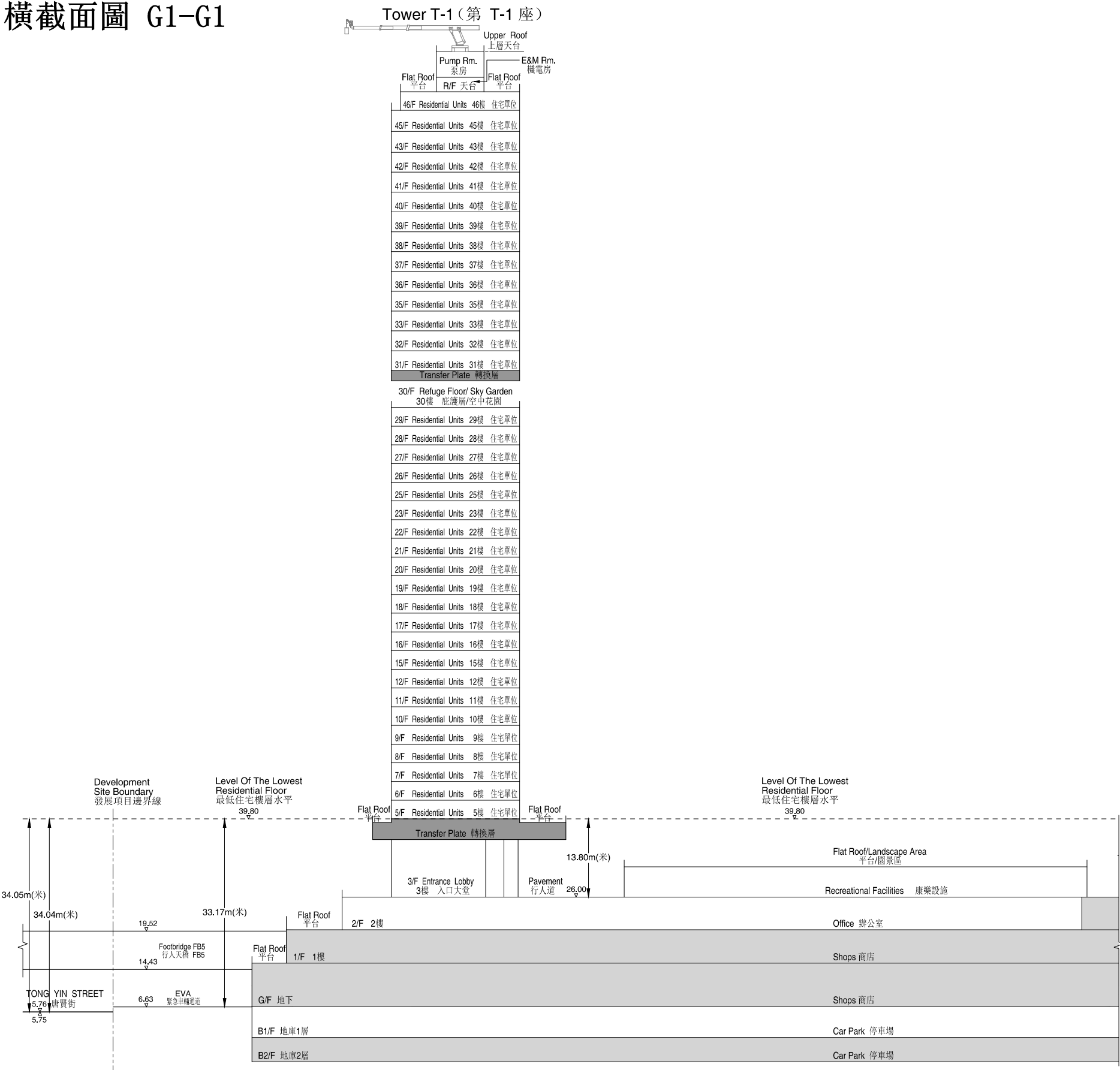
Development Site Boundary 發展項目邊界線
